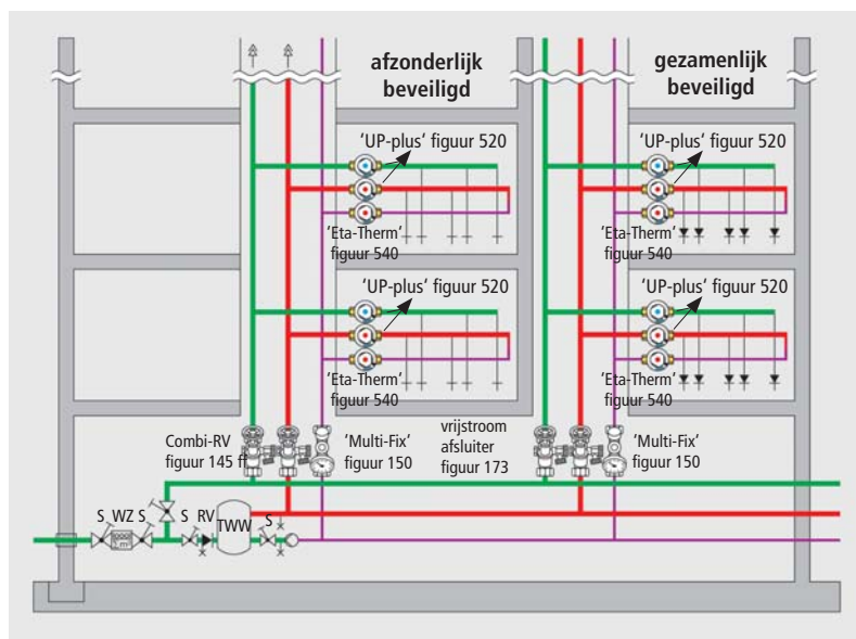
Installatieschema met verdieping circulatiesysteem met UP-regelventielen voor warmwater, warmwatercirculatie en koudwater
